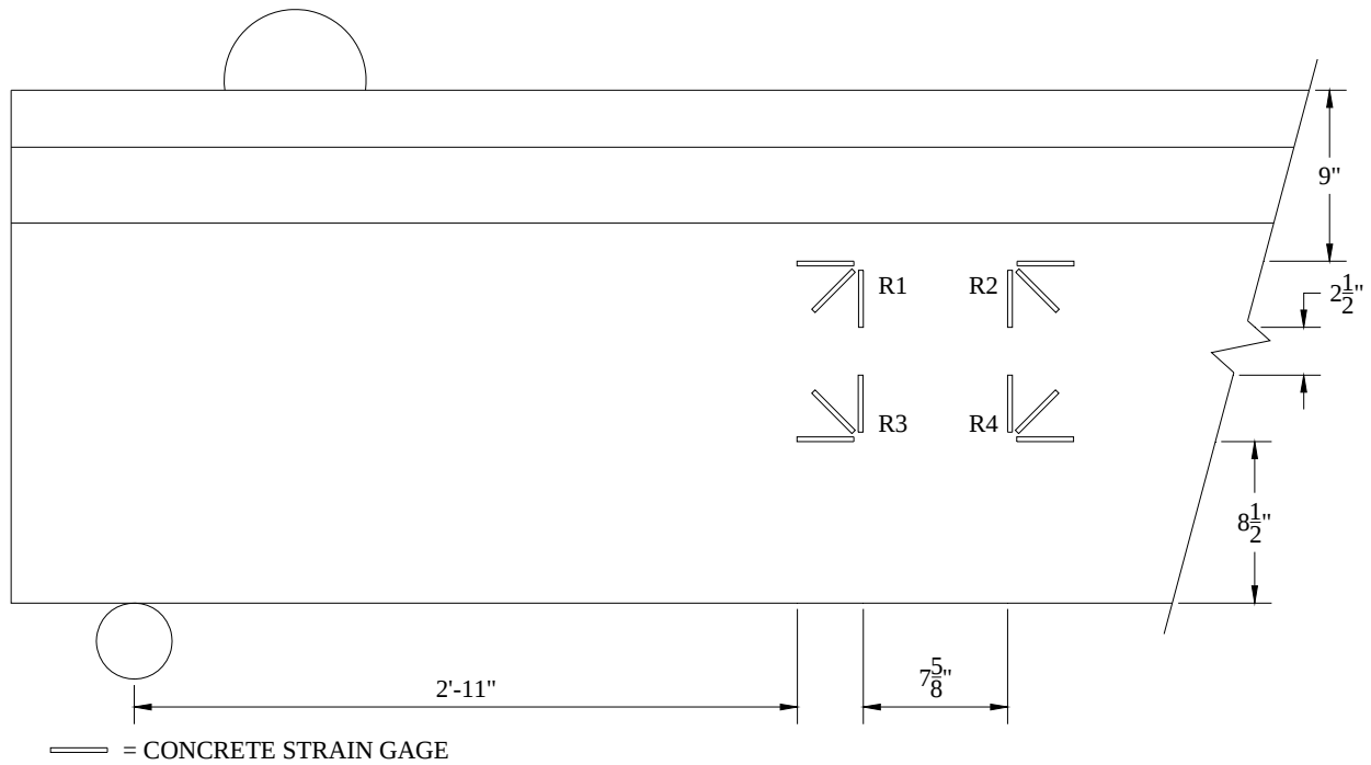
a. rosette positions
