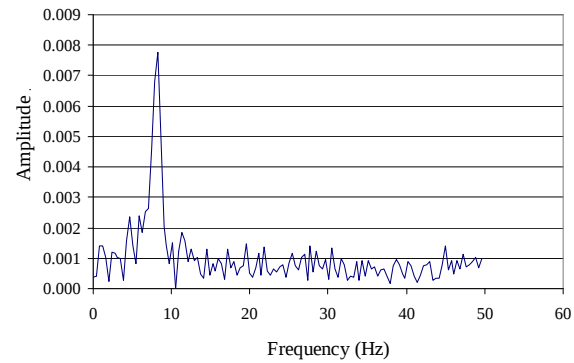
b. FFT; A3; 35mph
