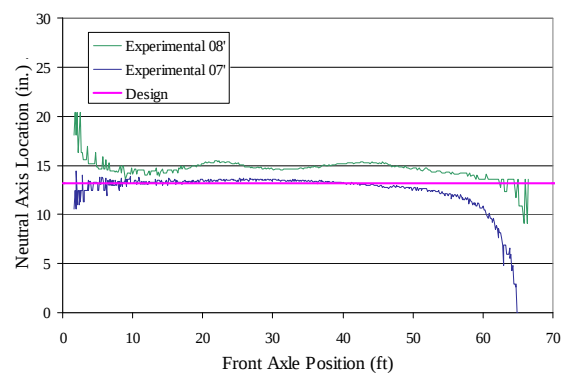
b. Girder G2, LC2
